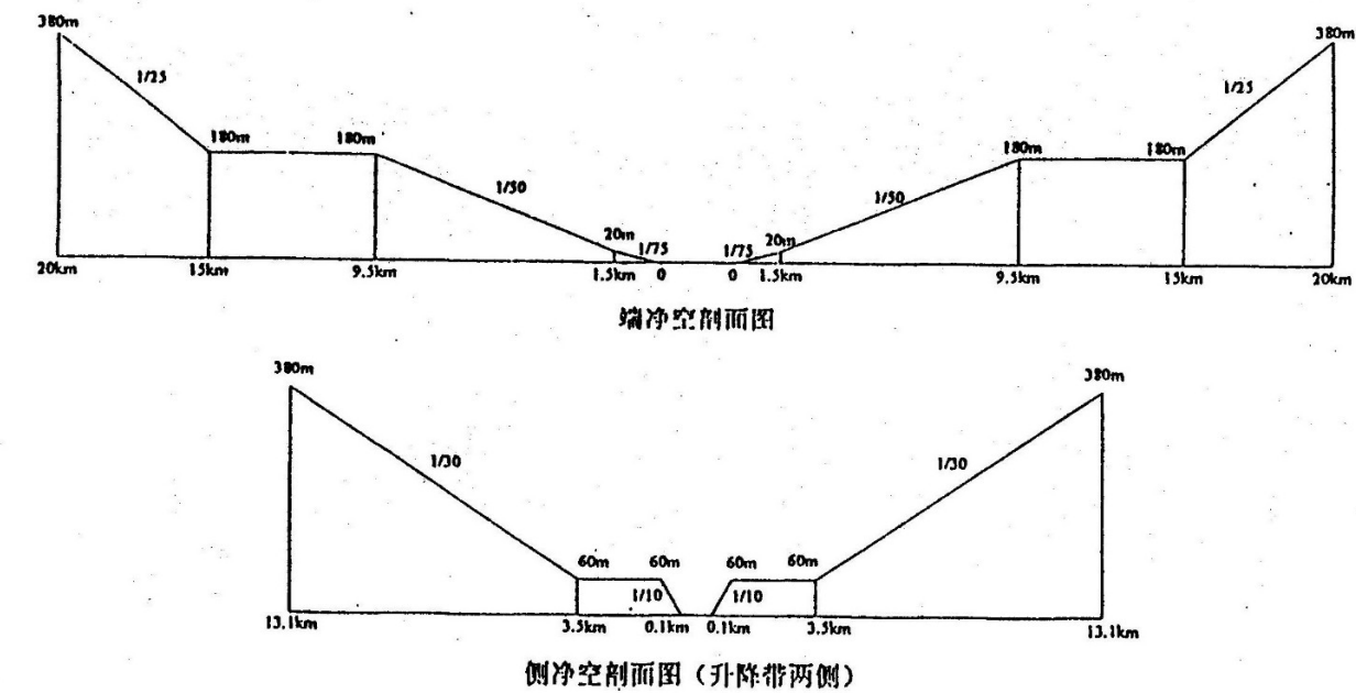
图 8-2 机场净空剖面示意图
