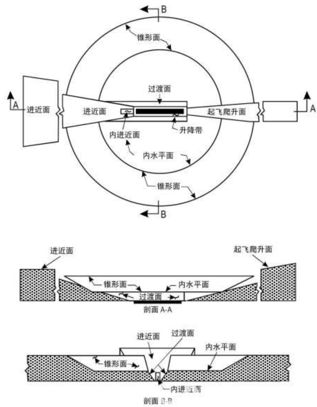
图 8-1 机场净空平面示意图
